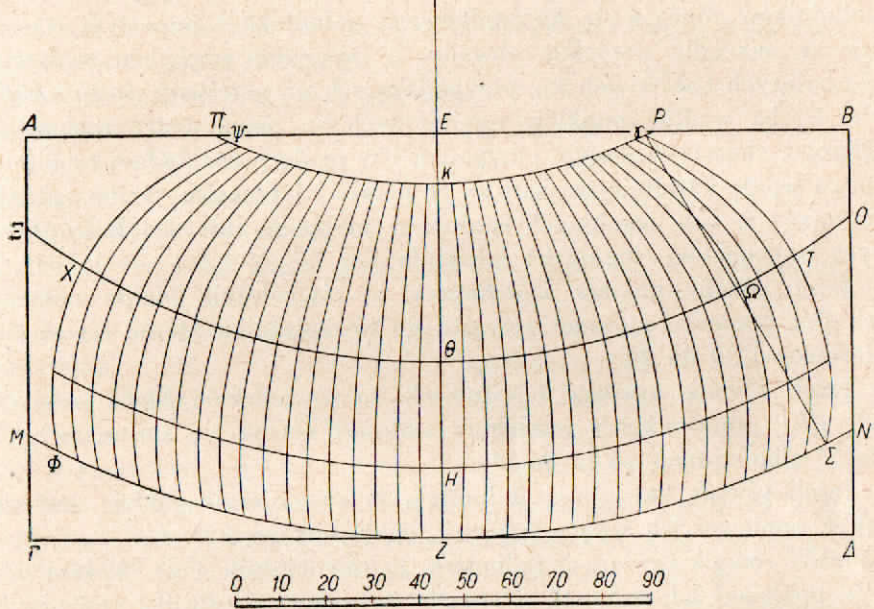
Ryc. 13. Rzut stereograficzny z południkami i równoleżnikami w kształcie łuków.
